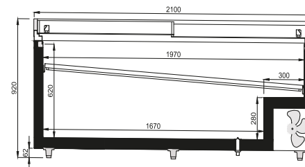
CORTE LONGITUDINAL
