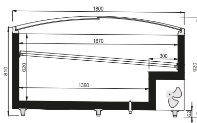
CORTE LONGITUDINAL
