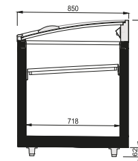
CORTE TRANSVERSAL
